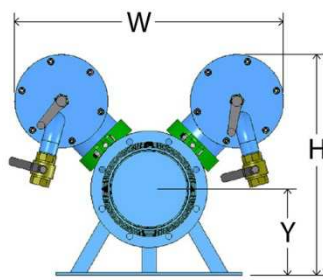
SA510B [2xSA506B]
